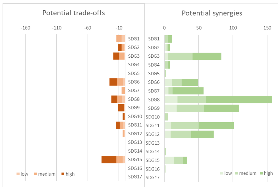
Слика 1: Синергии и компромиси меѓу Целите за одржлив развој и политиките и мерките во секторите за производство на електрична енергија и топлина, транспорт, згради и отпад
