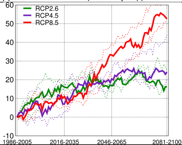
Должина на вегетациски период
