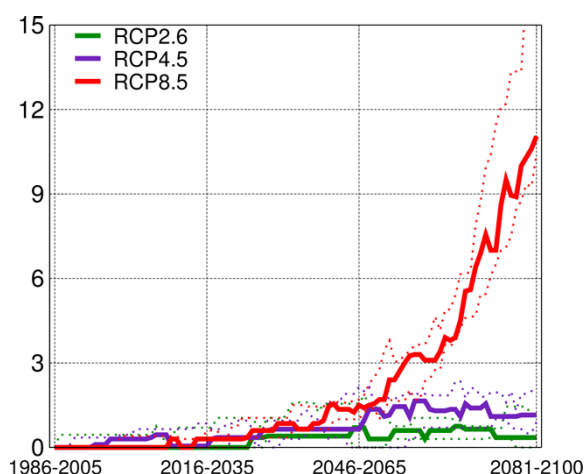
Сл. 6 Промени во траењето на топлотните бранови (во денови) за последователни 20-годишни периоди почнувајќи од 1986-2005 до 2081-2100, во однос на периодот 1986-2005, за сценаријата RCP2.6, RCP4.5 и RCP8.5. Полните линии се средна вредност на збир од повеќе избрани модели, а точкестите линии се збирен опсег од 25-тиот до 75-тиот перцентил.
